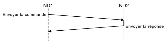
Figure C.1 – Communications de réponse à la commande
