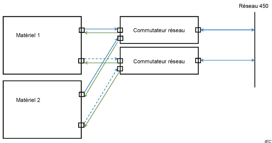
Figure G.4 – Exemple de deux matériels
