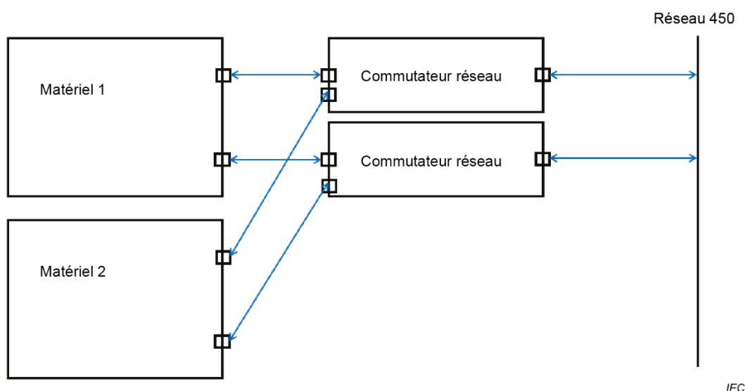
Figure G.2 – Exemple de deux matériels
