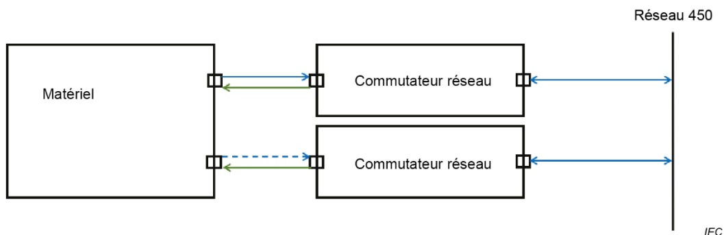
Figure G.3 – Deux interfaces réseau distinctes connectées à un seul et même réseau, mais une seule des interfaces réseau effectue les envois, à un moment donné
