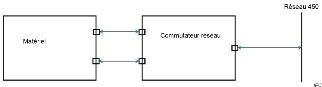
Figure G.5 – Deux interfaces réseau distinctes connectées à un seul et même réseau, mais un commutateur réseau permet de percevoir le matériel comme une seule interface
