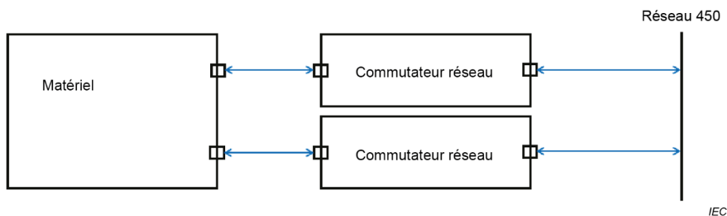
Figure G.1 – Deux interfaces réseau distinctes connectées à un seul et même réseau
