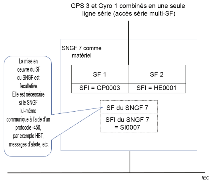
Figure 3 – Exemple de SNGF, accès série multi-SF
