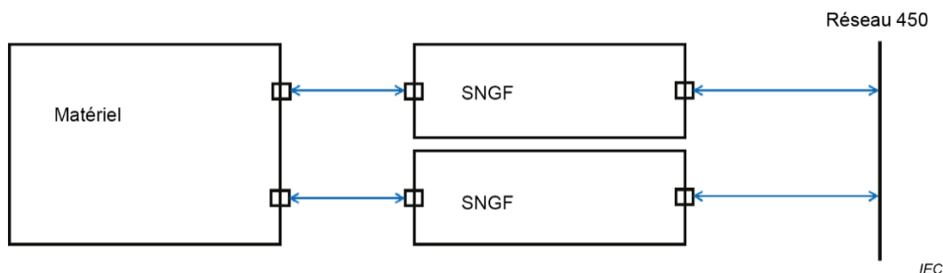
Figure G.7 – Un matériel avec deux interfaces série distinctes connectées au réseau par des SNGF distincts
